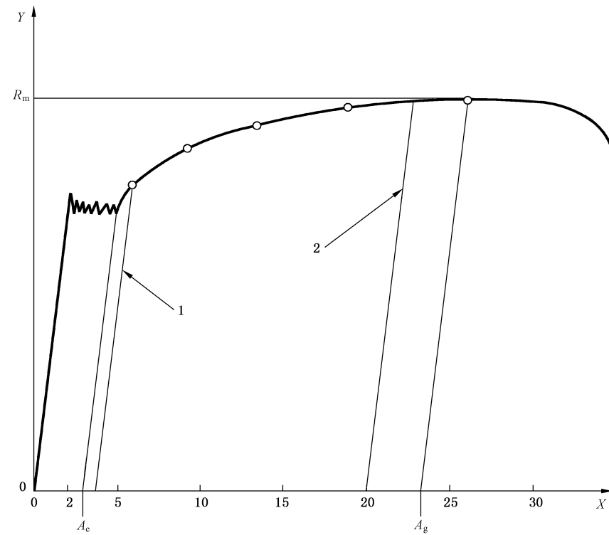
X—应变,%; Y—应力; 1—下限; 2—上限。
