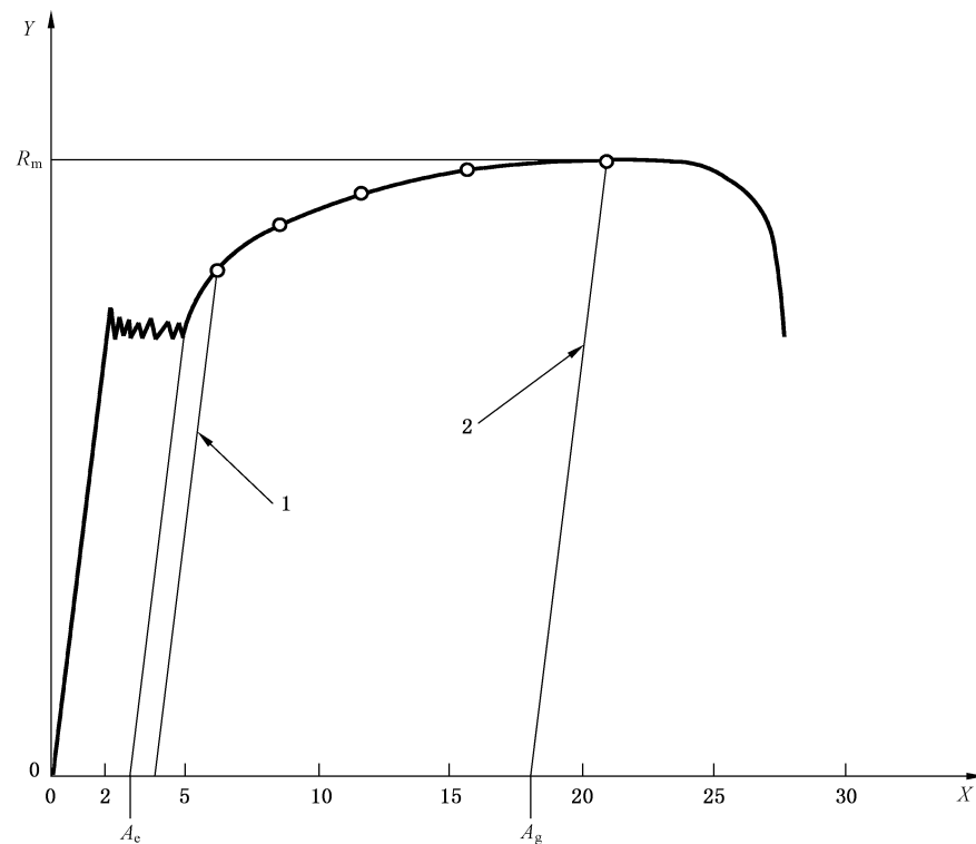
X—应变,%; Y—应力; 1—下限; 2—上限。
